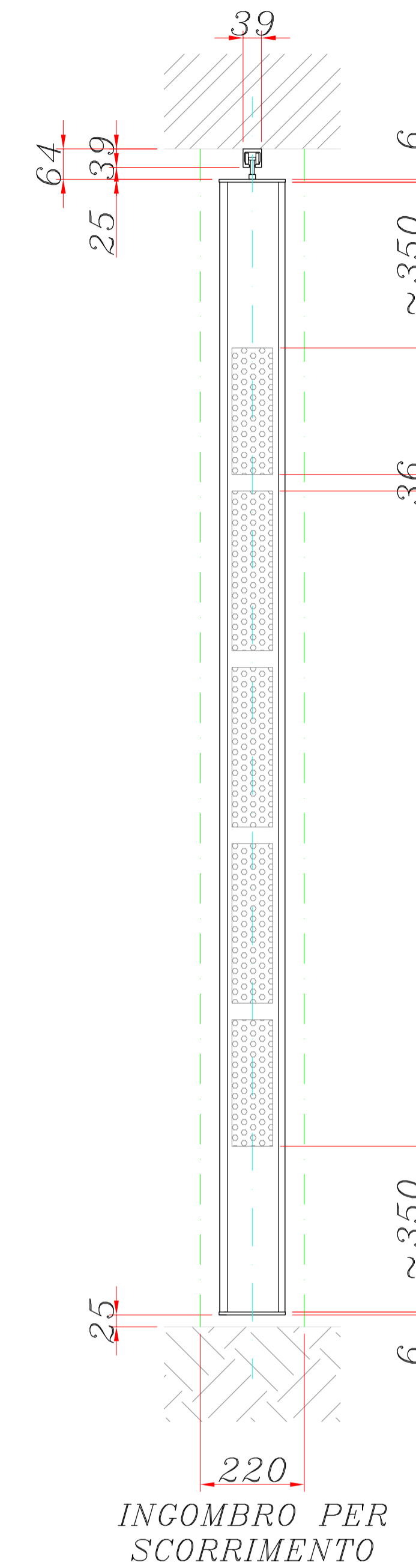
ELEMENTO WALL
