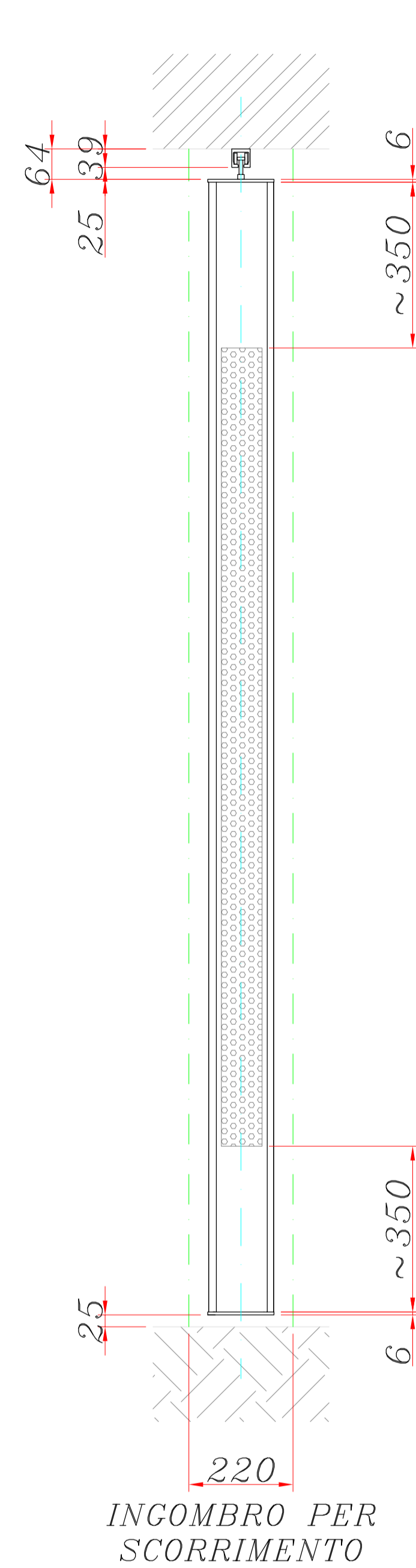
ELEMENTO MICROFORATO
