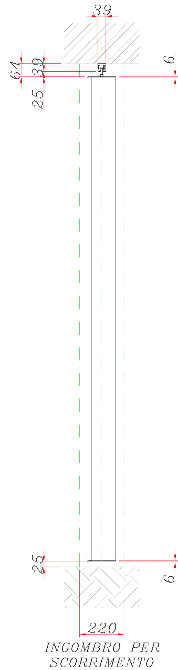
ELEMENTO CIECO
